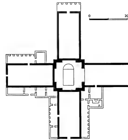
Antiocheia [1] am Orontes. St. Babylas, 379/380 n. Chr. (Grundriß).
